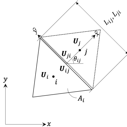
〈그림 2.1〉 Local Coordinate System (\hat{x}, \hat{y})
