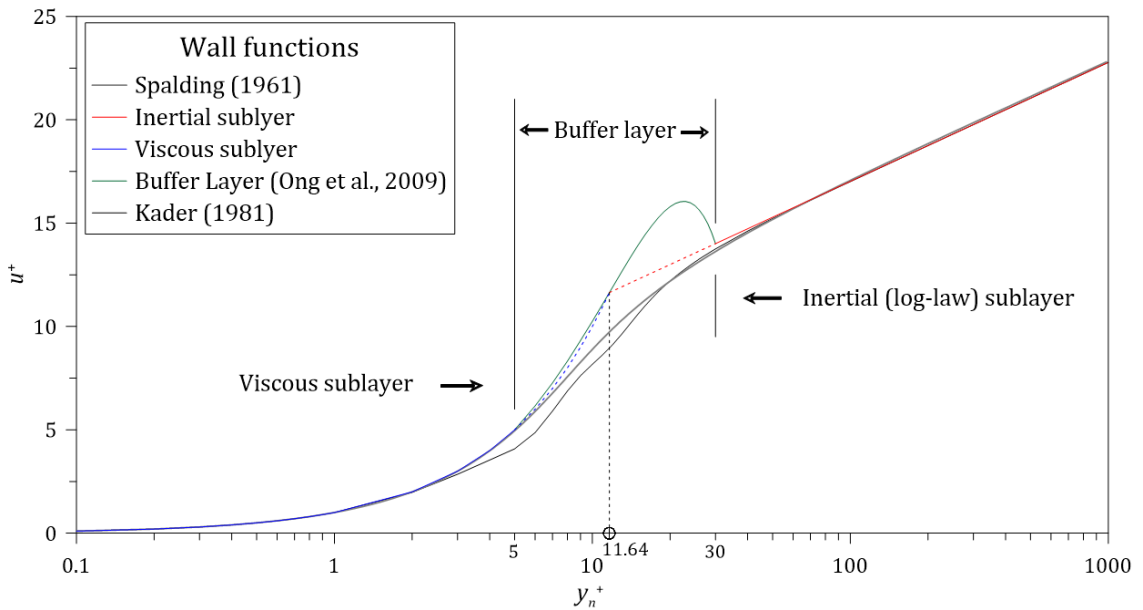
〈그림 F.1〉 Wall functions in turbulent boundary layer
